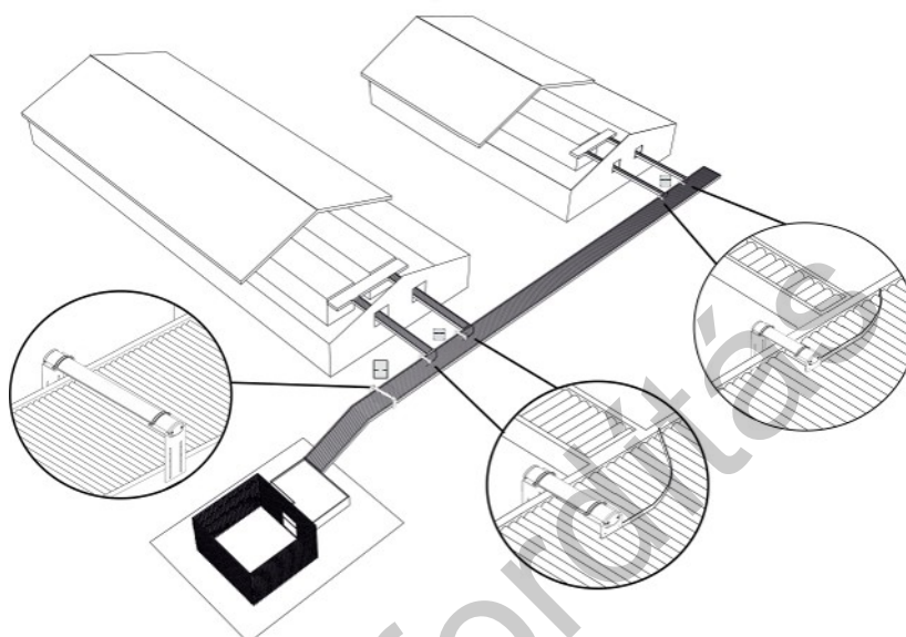
ábra 15: Az automatikus tojásszámláló elrendezésének vázlatos rajza.
