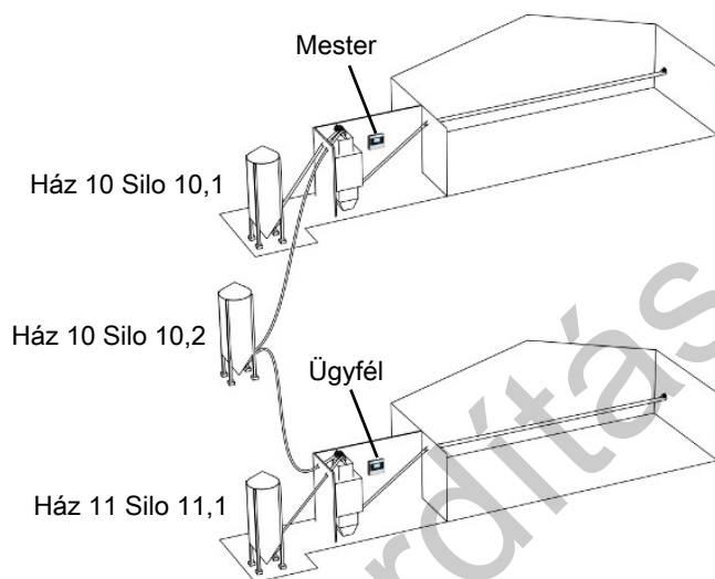
ábra 13: Példa a két ház között megosztott silóra a LAN-vezérlőkkel.
