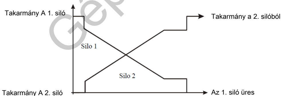
ábra 12: Amikor a siló tartalma eléri a beállított mennyiséget, megkezdődik a fokozatos átmenet egy másik silóra.
