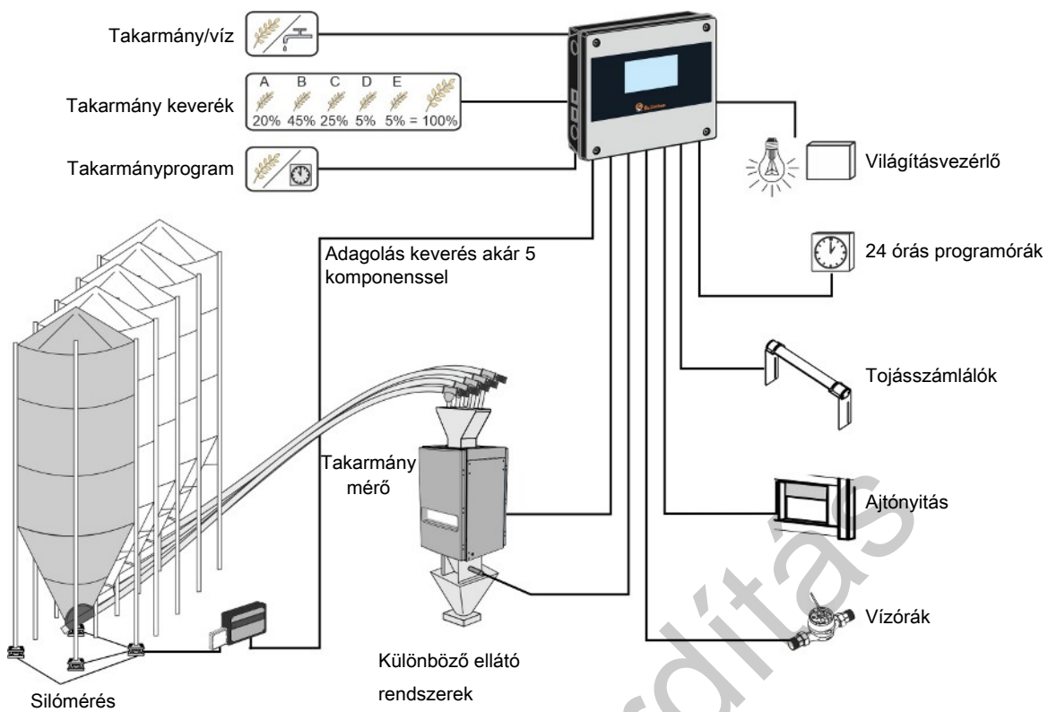
ábra 5: Példa a csatlakozási lehetőségekre.
