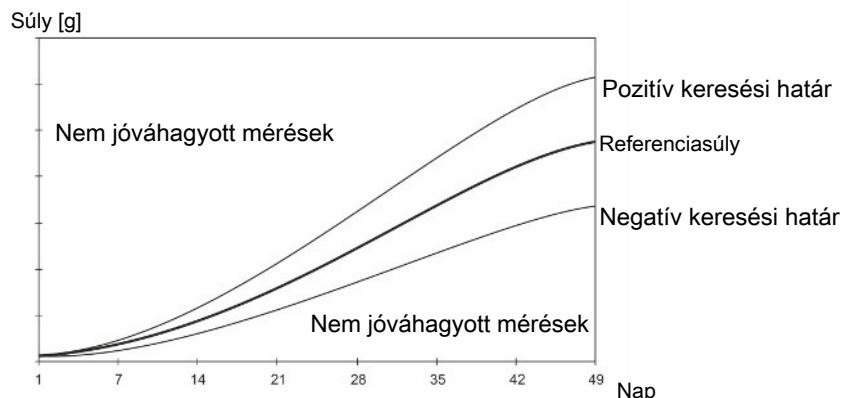
ábra 6: Példa a keresési korlátozásra a referenciatömeghez viszonyítva. Ha a vezérlőben az állattípus kakasokra és tojókra van állítva, a keresési határhoz viszonyítva pozitív és a negatív beállítást lehet alkalmazni.
